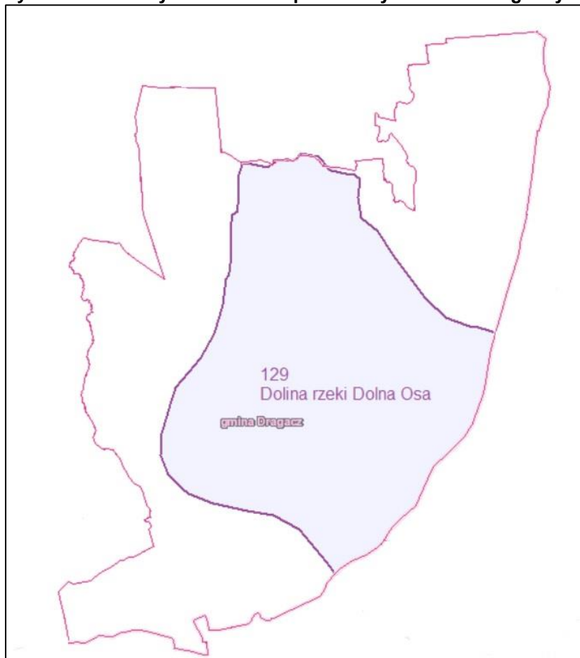
Rysunek 6 Główny zbiornik wód podziemnych na terenie gminy Dragacz
